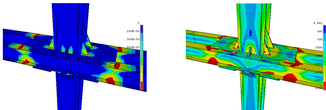
شکل ۱۱: توزیع تنش فون میسزو کرنش پلاستیک معادل در زاویه دریفت 0.3^\circ در بارگذاری سیکلی، مدل KHV01 [۲]
