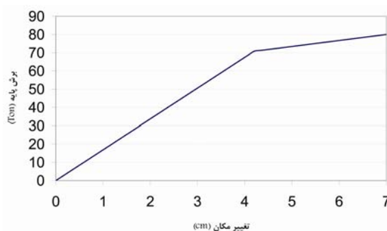
شکل ۱۲: نمایش منحنی ظرفیت سیستم مهاربند مقاوم در برابر کماتش در سطح خطر ۲
