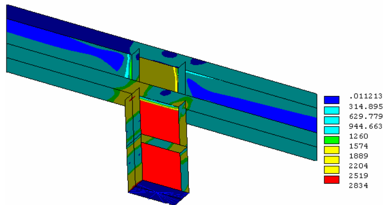
شکل ۵- کانتور نوعی تنش معادل فون میسز برای چهار نمونه اول
