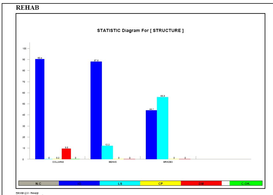
شکل ۶-نمایش گرافیکی حاصل از ارزیابی سازه
