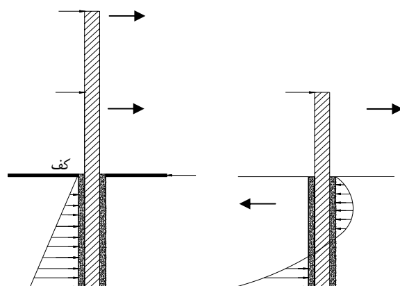
ب) ساختمان دو یا سه طبقه
