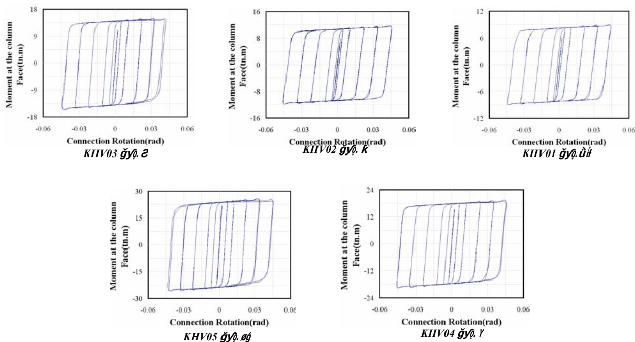
شکل ۱۹. منحنی‌های لنگر چرخش اتصال [۲]
