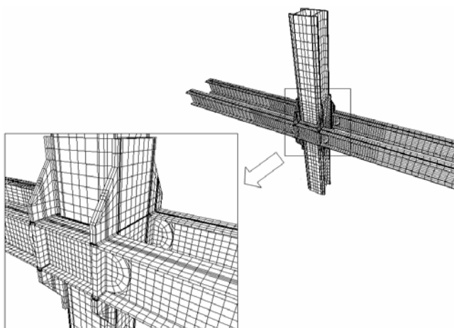
شکل ۹: نمونه‌ای از مش‌بندی مدل‌های اجزای محدود [۲]
