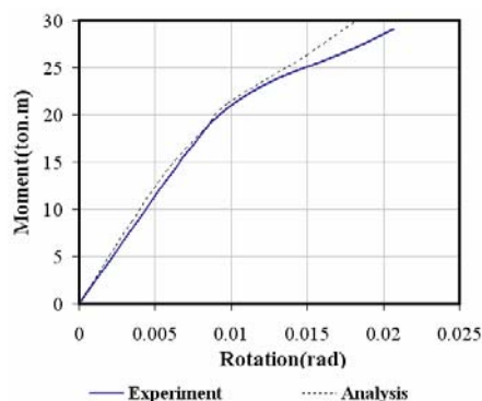
شکل ۶: مقایسه پوش حاصل از منحنی‌های ممان-دوران نمونه آزمایشگاهی و مدل اجزای محدود [۲]
