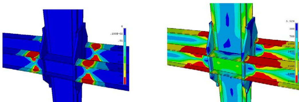
شکل ۱۱: توزیع تنش فون میسزو کرنش پلاستیک معادل در زاویه دریفت ۰/۵+ رادیان در بارگذاری سیکلی، مدل KHV01 [۲]
