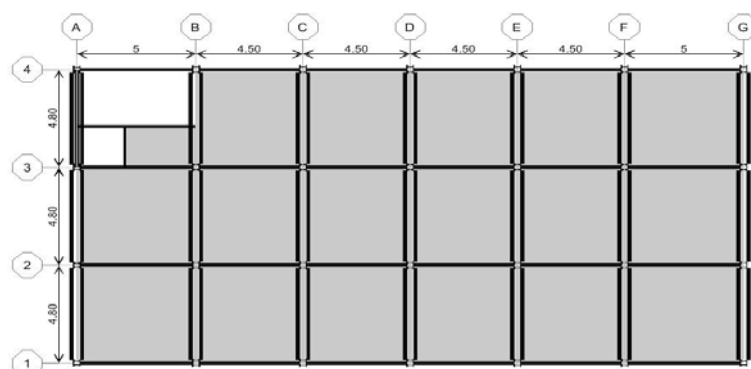
پلان ساختمان شماره ۳
