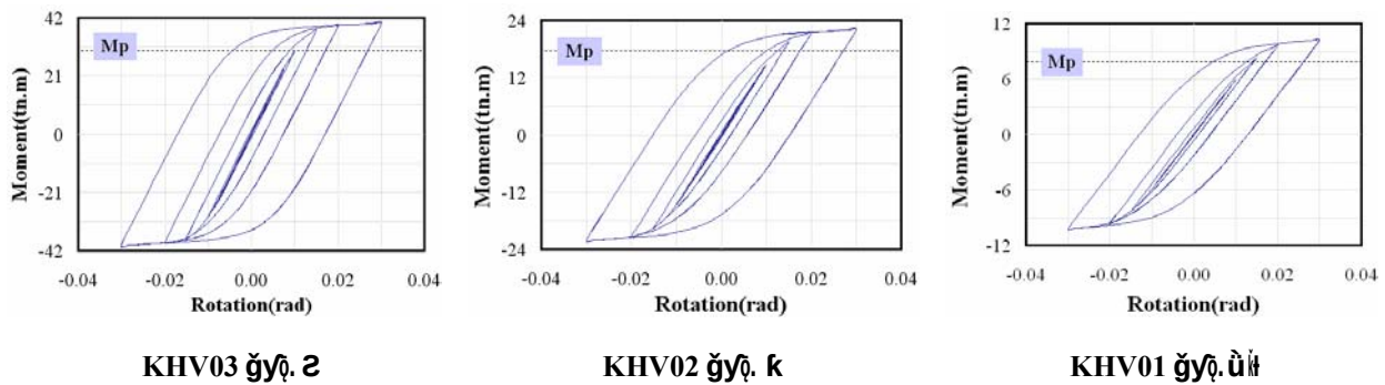
شکل ۱۴: منحنی‌های هیستریزیس ممان - دوران [۲]
