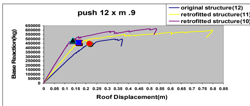
نمودار ۱۱- منحنی ظرفیت ساختمان ۱۲ طبقه قبل و بعد از تقویت (در جهت X)
