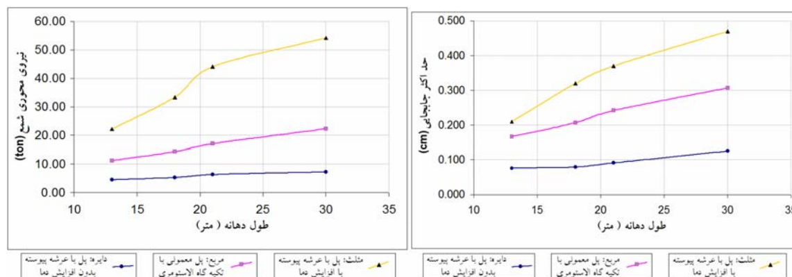
شکل - نتایج آنالیز با مدل خاک خطی (قسمت اول)
