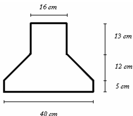
شکل ۲: ابعاد ورق گیرداری نمونه آزمایشگاهی [۶]
