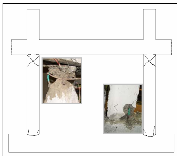
شکل ۵: الگوی ترک خوردگی در قاب‌های بدون میانقاب
