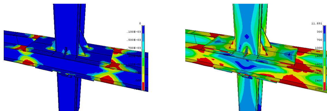
شکل ۱۳: توزیع تنش فون میسزو کرنش پلاستیک معادل در زاویه دریفت 0.3^\circ در بارگذاری سیکلی، مدل KHV03 [۲]
