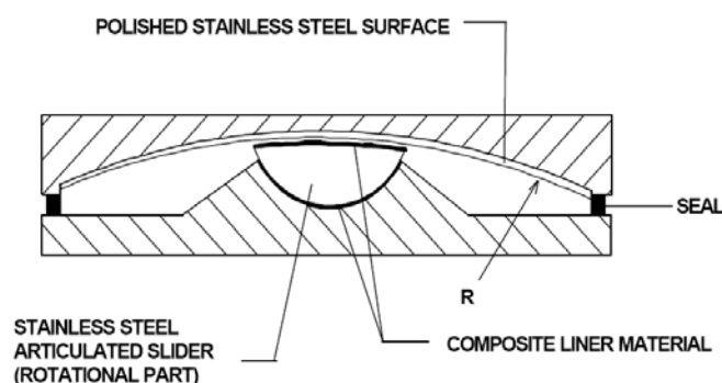
شکل - سیستم جداسازی آونگ اصطکاکی
