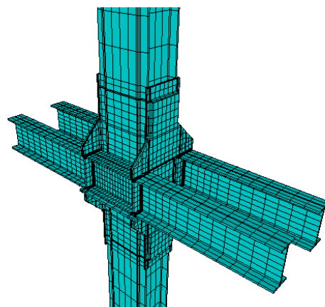
شکل ۳: مدل اجزای محدود نمونه آزمایشگاهی
