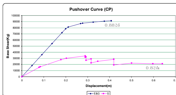
نمودار (۲): نمودار برش پایه-تغییر مکان دو قاب شش طبقه در سطح زلزله طراحی ۲٪ در ۵۰ سال
