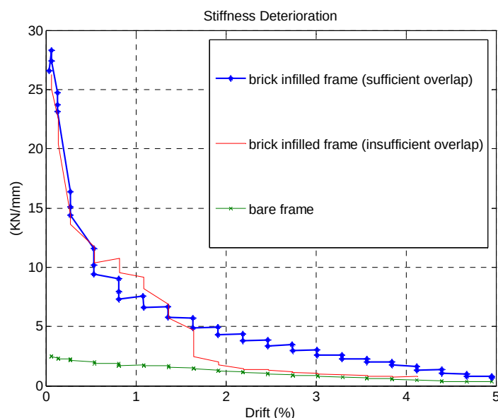
شکل 10: منحنی تغییرات سختی در نمونه‌های مختلف
