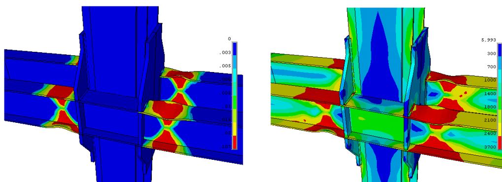
شکل ۱۵: توزیع تنش فون میسزو کرنش پلاستیک معادل در زاویه دریفت ۰/۰۵ رادیان در بارگذاری سیکلی، مدل KHV05 [۲]
