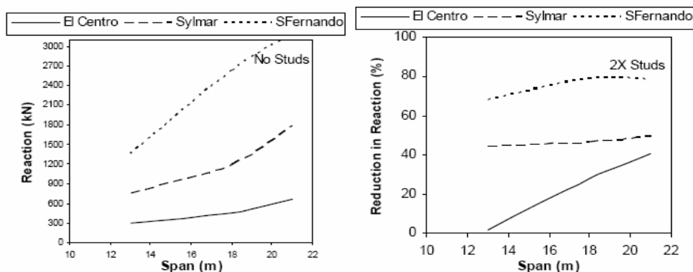
شکل : کاهش نیروی وارده به زیر سازه با استفاده از دستگاه
