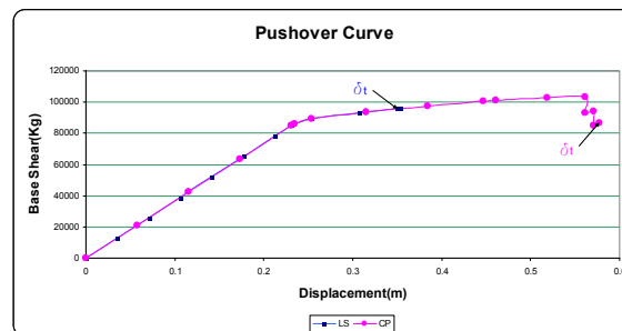
نمودار (۳): نمودار برش پایه-تغییر مکان دو قاب هشت طبقه در سطح زلزله طراحی ۲٪ در ۵۰ سال
