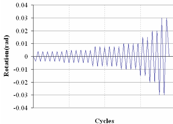
شکل ۱۰: بارگذاری سیکلی اعمالی به نمونه‌ها
