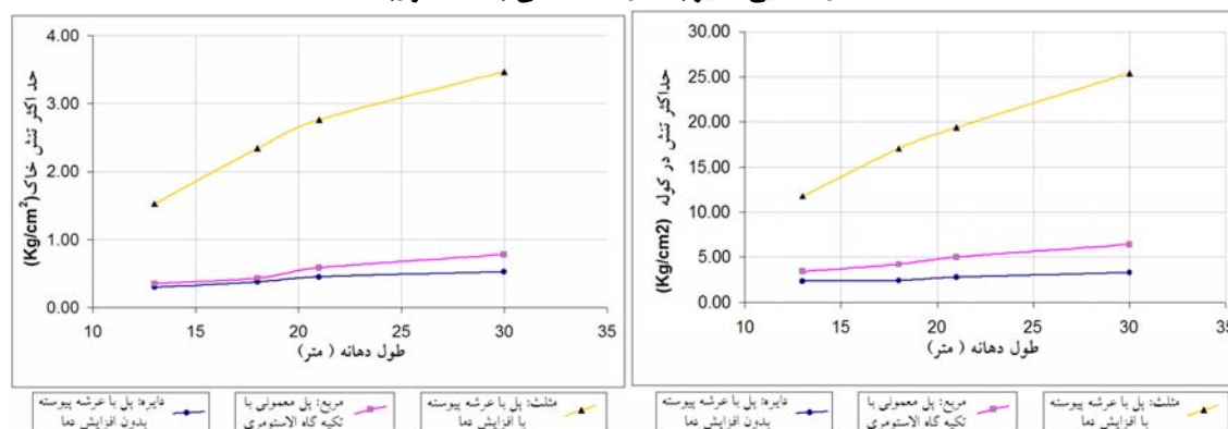
شکل ۳ نتایج آنالیز با مدل خاک خطی (قسمت دوم)
