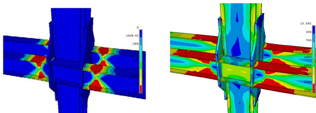
شکل ۱۲: توزیع تنش فون میسزو کرنش پلاستیک معادل در زاویه دریفت ۰/۵+ رادیان در بارگذاری سیکلی، مدل KHV02 [۲]
