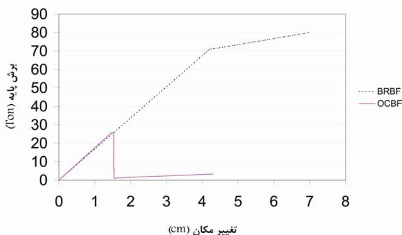
شکل ۱۴: مقایسه منحنی ظرفیت سیستم مهاربند مقاوم در برابر کمانش و مهاربند هم مرکز معمولی
