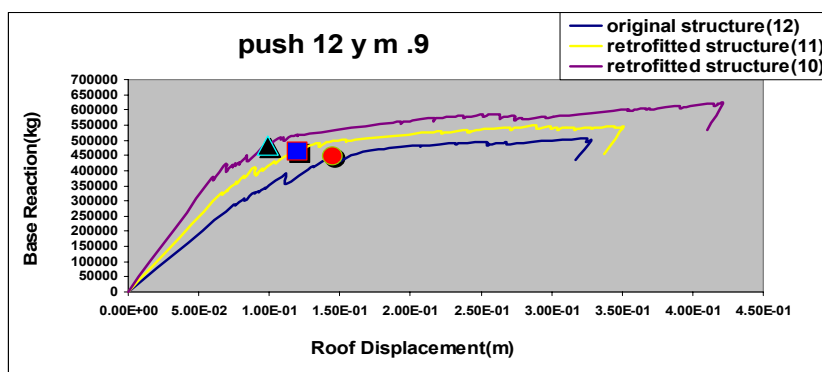
نمودار ۱۳- منحنی ظرفیت ساختمان ۱۲ طبقه قبل و بعد از تقویت (در جهت Y)
