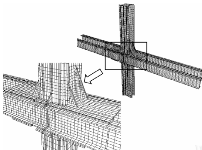
شکل ۹: نمونه‌ای از مش‌بندی مدل‌های اجزای محدود [۲]
