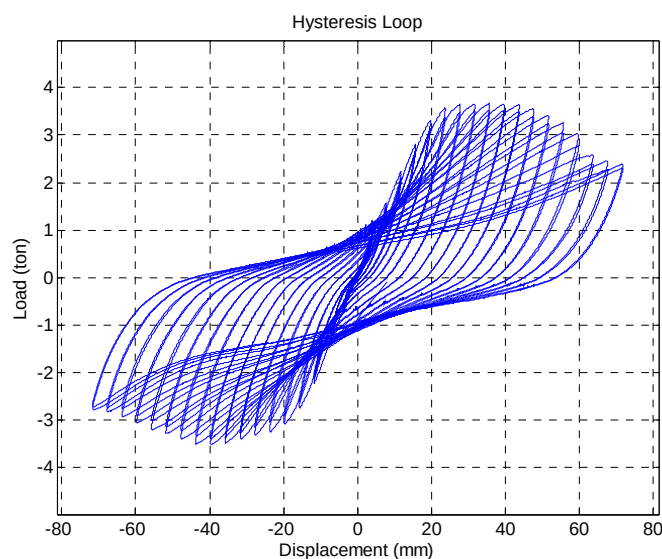
شکل 7: منحنی رفتاری قاب بدون میانقاب
