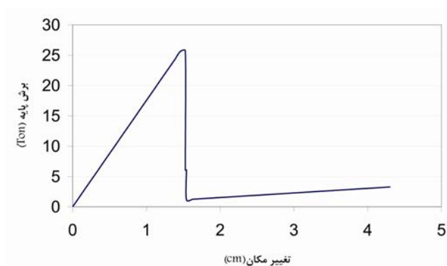
شکل ۸: منحنی ظرفیت سیستم قاب بندی شد هم مرکز معمولی
