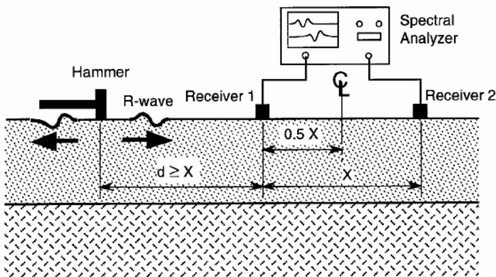
شکل (۳-۱): نحوه عملکرد روش تحلیل طیفی امواج (SASW)
