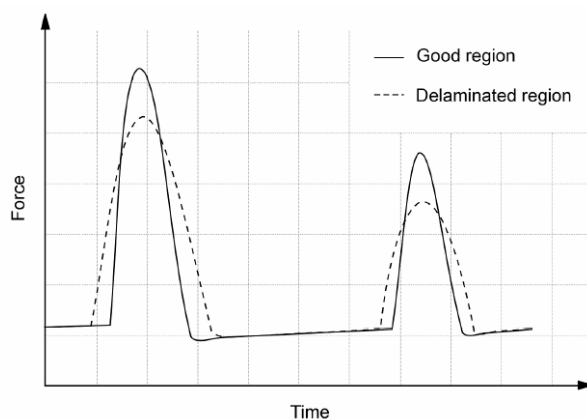
شکل ۱: تاریخچه زمانی نیرو در آزمایش ضربه صوتی
