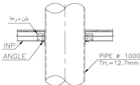
شکل ۵: جزئیات اتصال سیستم مقاوم ساز در تراز طبقات
