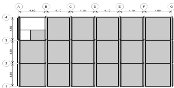
پلان ساختمان شماره ۲
