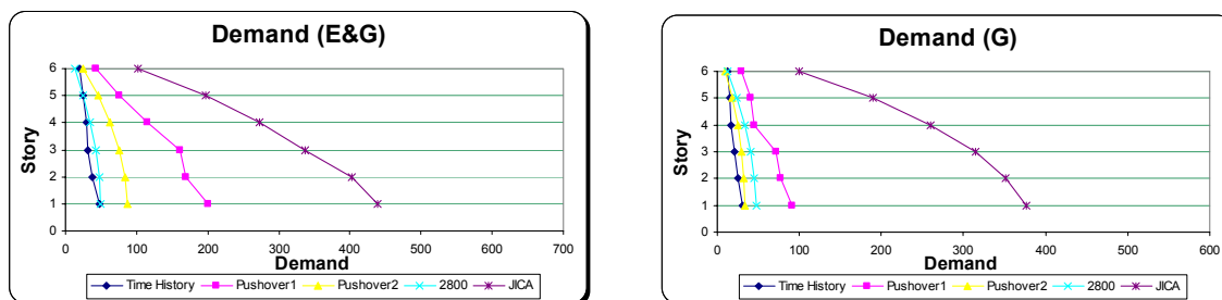
نمودار(۵): به ترتیب نمودار مقایسه‌ای تقاضای قاب شش طبقه G و E&G در سطح زلزله طراحی ۱۰٪ در ۵۰ سال
