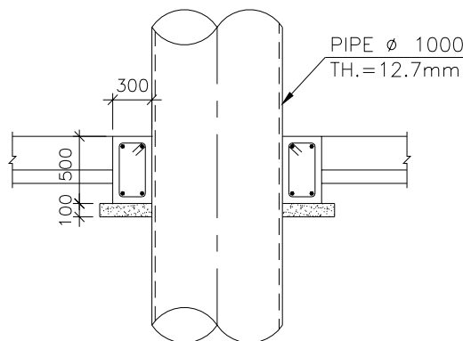
شکل ۶: جزئیات اتصال سیستم مقاوم ساز به کف
