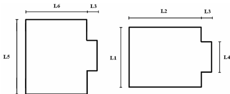
شکل ۸: ابعاد ورق گیرداری قائم [۴]
