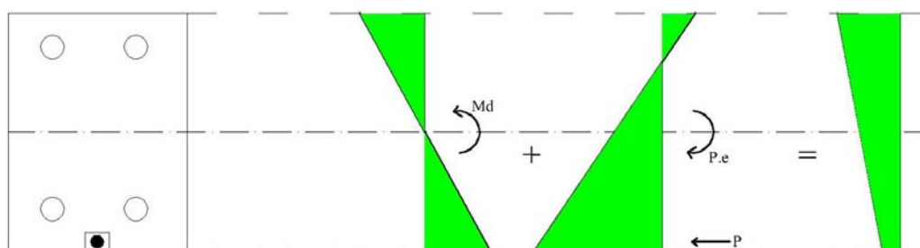
شکل ۲- توزیع تنش در یک مقطع پیش‌تنیده [۱۳]
