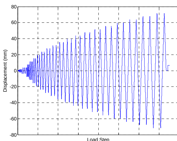
شکل 3: تاریخچه بارگذاری نمونه‌ها
