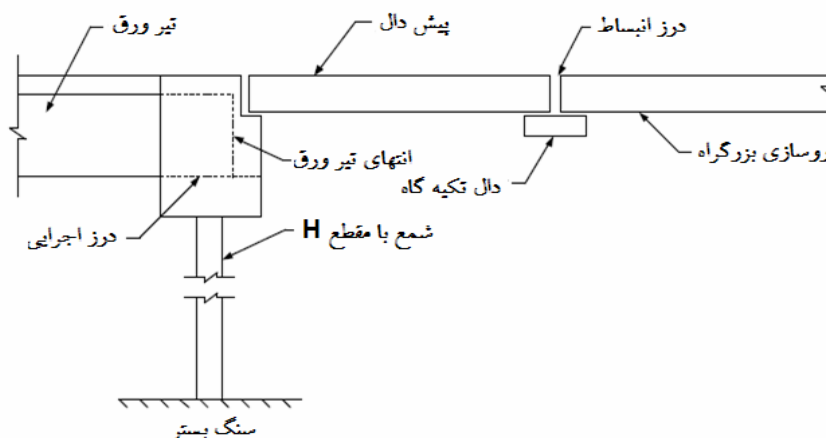
شکل- شکل کلی کوله یکپارچه و شمع و پیش دال و پی زیر پیش دال
