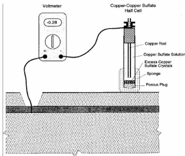
شکل (۷-۱): نمای کلی روش پتانسیل نیم سلولی
