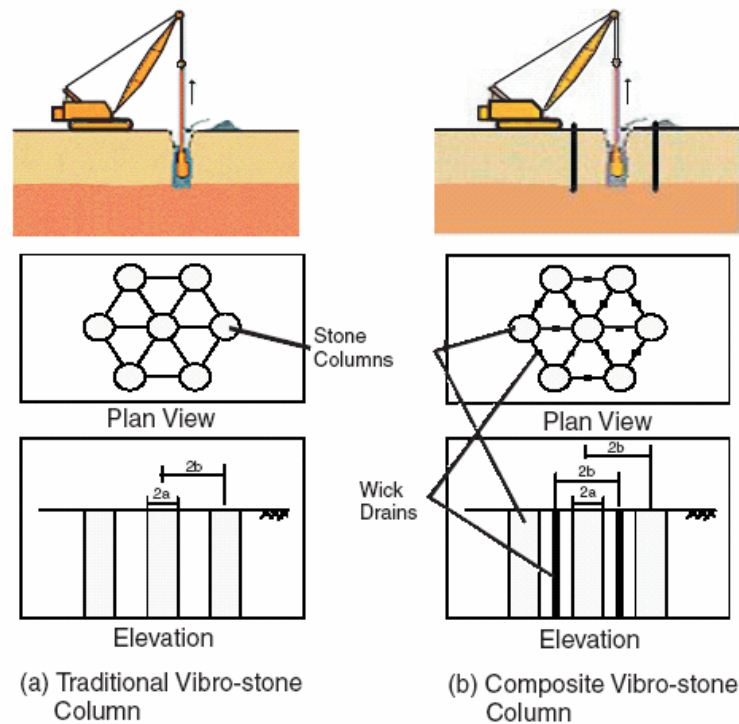
شکل ۲-۱. اجرای سنتی و جدید روش ستون سنگی
