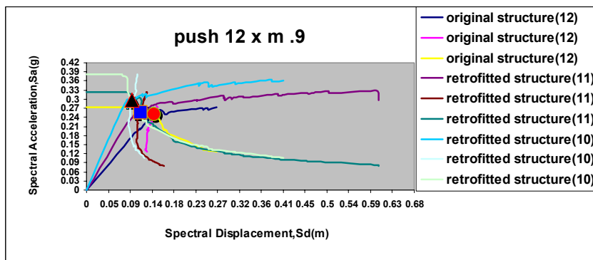
نمودار ۱۲- منحنی های ظرفیت و نیاز طیفی ساختمان ۱۲ طبقه قبل و بعد از تقویت (نقطه هدف X)
