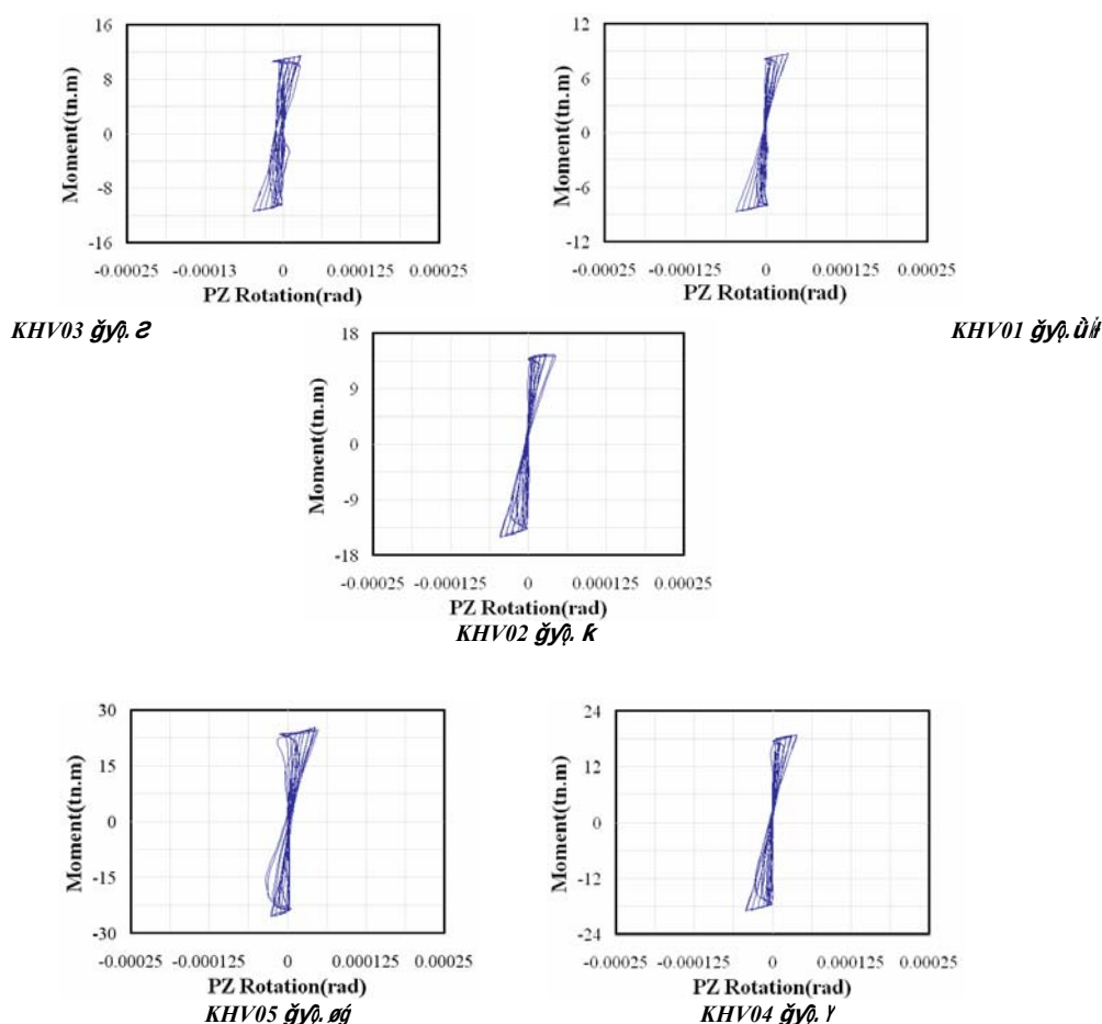
شکل ۱۸: منحنی های لنگر- زاویه چرخش چشمه اتصال [۲]
