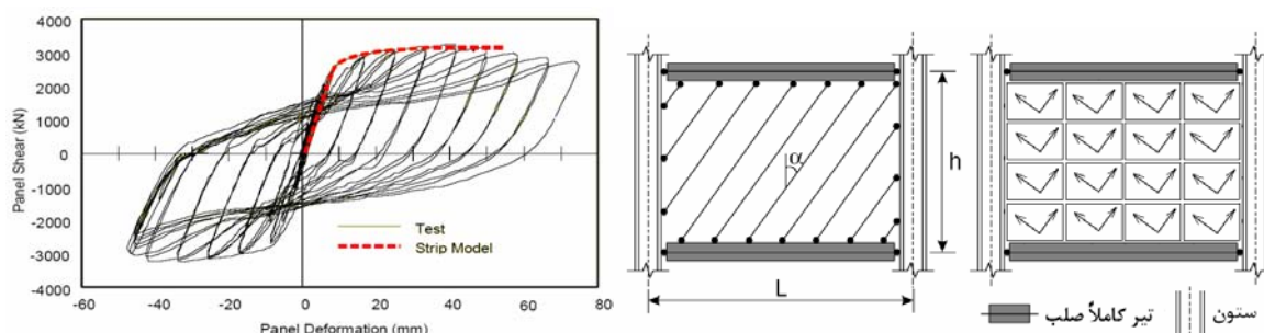
شکل ۷: مدل پوسته Anisotropic و مدل نواری [۱] [۶] و مقایسه رفتار آزمایشگاهی با نتایج مدل نواری [۴]
