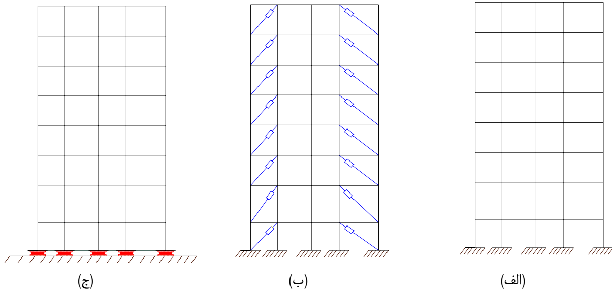
شکل (۶): قاب مقاوم‌سازی شده با روش الف (تقویت اعضا، ب) نصب میراگر، ج) جداسازی لرزه‌ای
