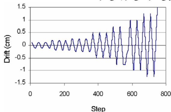
شکل ۳- بارگذاری تناوبی مطابق با پیشنهاد SAC-ATC 24
