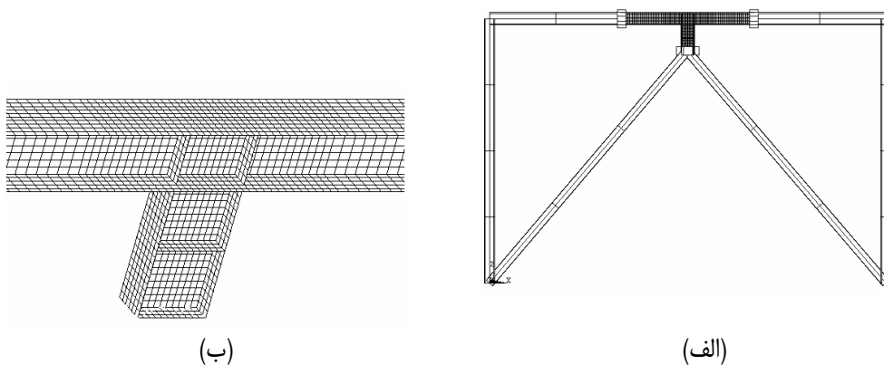
شکل ۲- نمونه‌ای از مش‌بندی اجزاء محدود قاب‌ها: (الف) مدل کلی؛ (ب) مش‌بندی پانل برشی و نواحی مجاور آن
