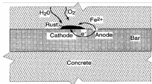
شکل (۱-۶): خوردگی آرماتور فولادی احاطه شده توسط بتن (آهن در محیط آند حل شده و به عنوان زنگار کاتد ته نشین می‌شود).
