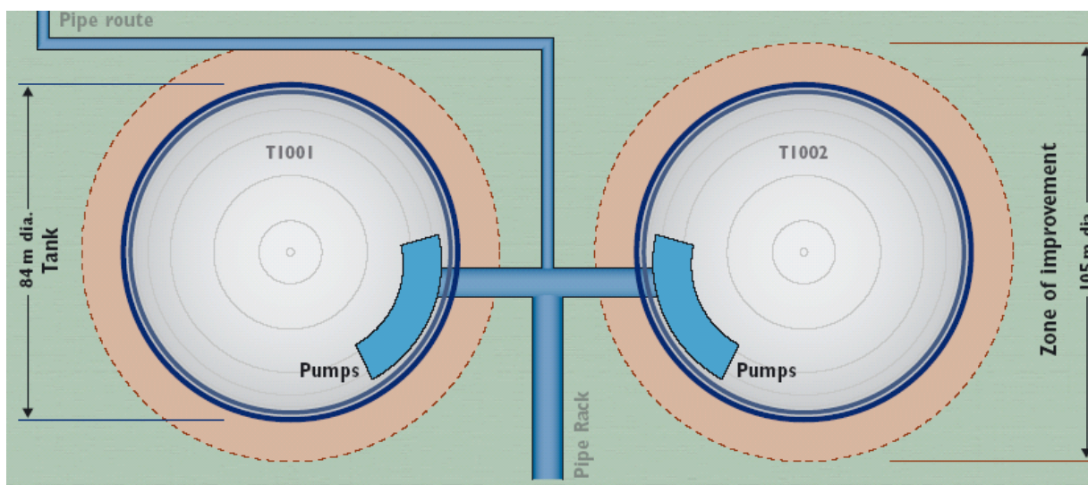
شکل ۵-۳. پلان مخازن و فونداسیون تحت بهسازی
