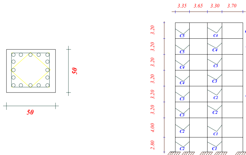
شکل (۲): مقطع C1
