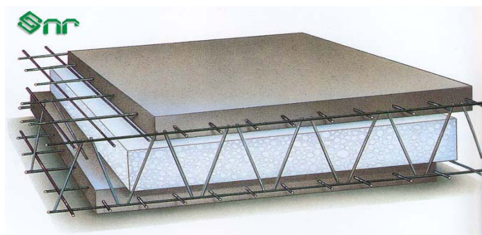
شکل ۱- پانل ساندویچی شاتکریتی
