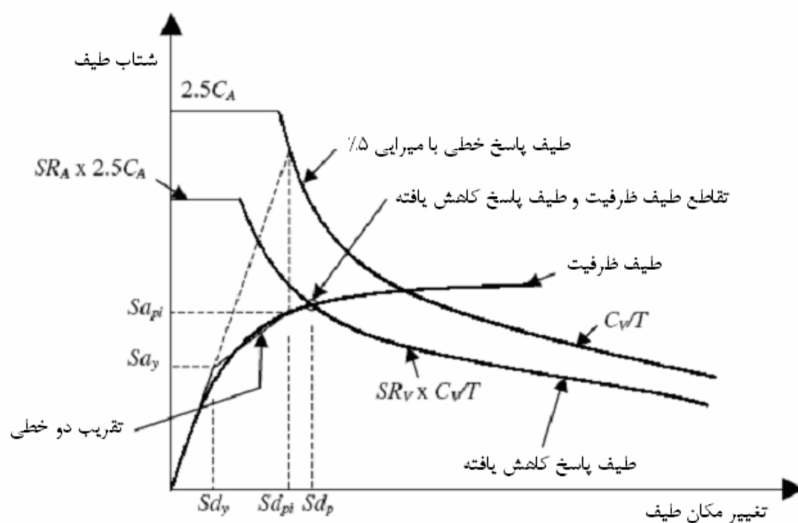
شکل ۲: تعیین نقطه عملکرد سازه در تحلیل Push Over [۱۰]
