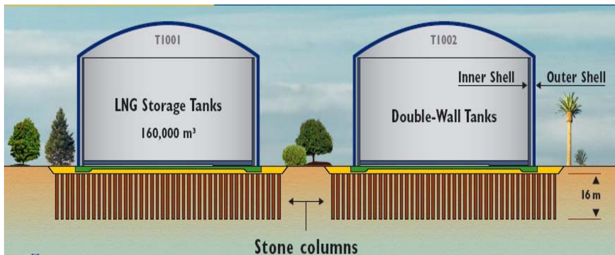
شکل ۵-۲. پروفیل مخازن و محل قرارگیری ستونها
