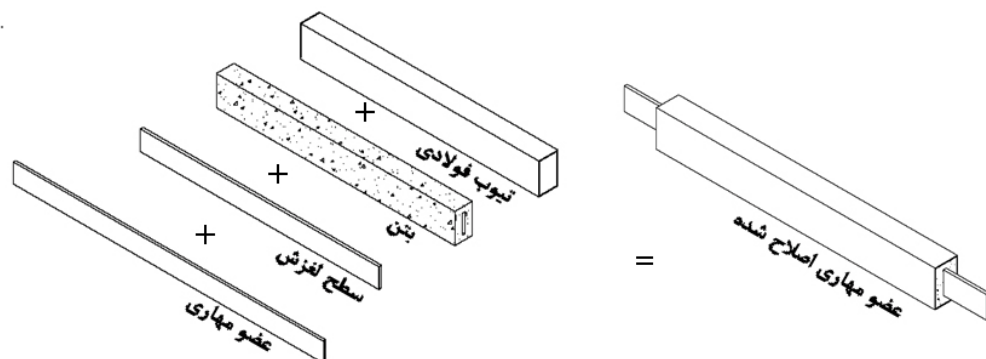
شکل ۲: طرح شماتیک مهاربندی‌های مقاوم در برابر کماتش [۶]
