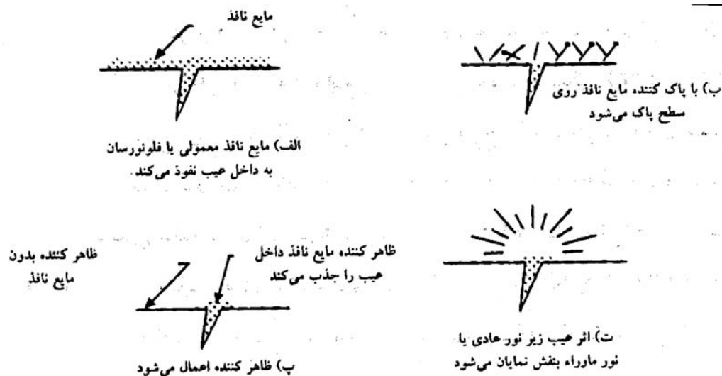
شکل (۲-۱): مراحل مختلف انجام آزمایش مايع نافذ
