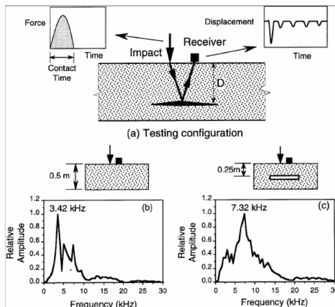
شکل (۲-۱) (a) نحوه عملکرد روش انعکاس ضربه، (b) طیف دامنه ارتعاش برای آزمایش دال بدون نقص، (c) طیف دامنه ارتعاش برای آزمایش دال توخالی
