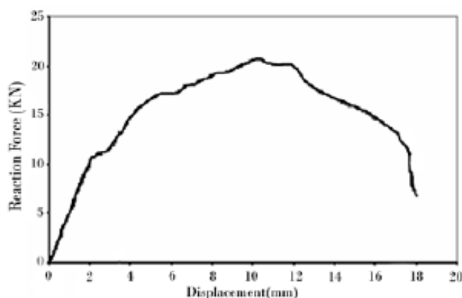
۶- نمودار پوش بار - تغییر مکان دیوار تنها [8]
