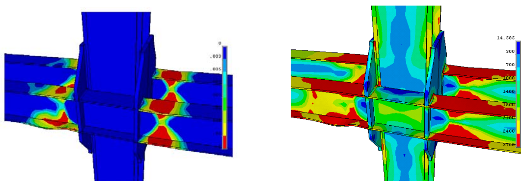
شکل ۱۳: توزیع تنش فون میسزو کرنش پلاستیک معادل در زاویه دریفت ۰/۵+ رادیان در بارگذاری سیکلی، مدل KHV03 [۲]
