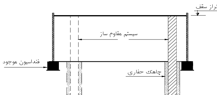
شکل ۳: سیستم سازه‌ای بهسازی لرزه‌ای نوین در ارتفاع یک ساختمان یک طبقه
