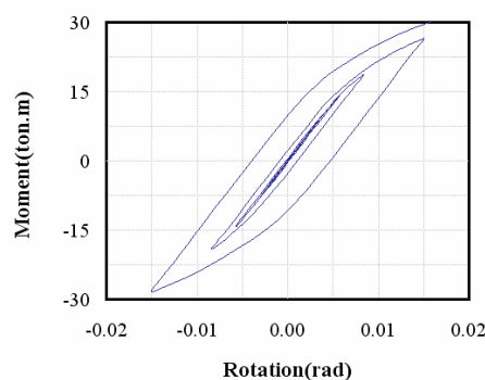
شکل ۵: منحنی چرخه‌ای ممان-دوران مدل اجزای محدود نمونه آزمایشگاهی [۲]
