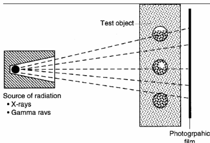
شکل (۴-۱): نحوه عملکرد روش رادیوگرافی در تعیین محل آرماتورها و حفره‌های مجاری پیش تنیده
