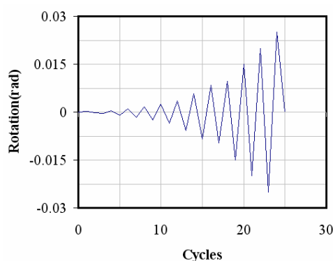
شکل ۴: دوران اعمالی به اتصال ساخته شده در مرکز تحقیقات مسکن [۶]
