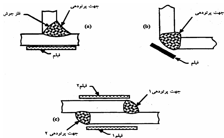
شکل (۳-۲): رادیوگرافی از جوش‌های گوشه
