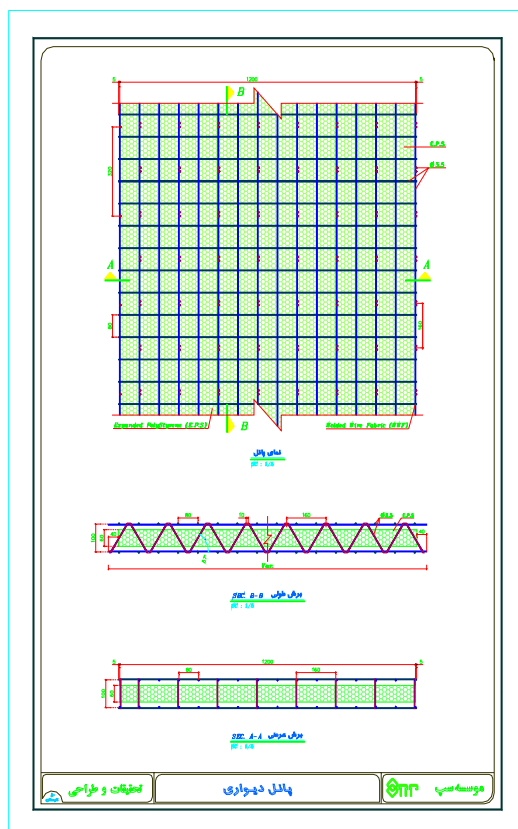
شکل ۲- مشخصات پانل دیواری
