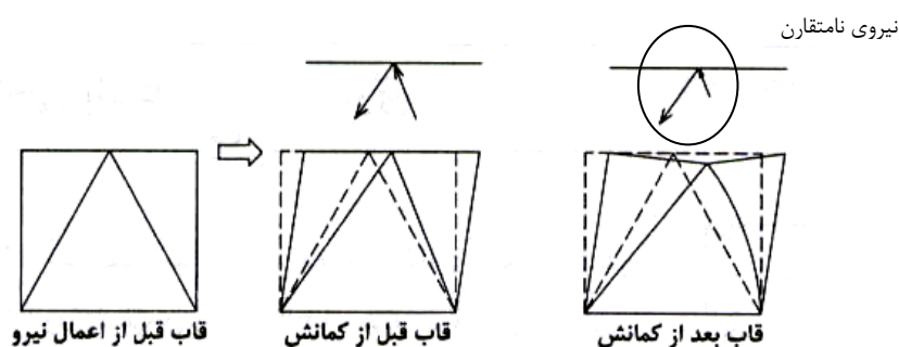
شكل ۱: ايجاد نيروى نامتقارن در تير طبقه بادبندى‌هاى شورون [۵]
