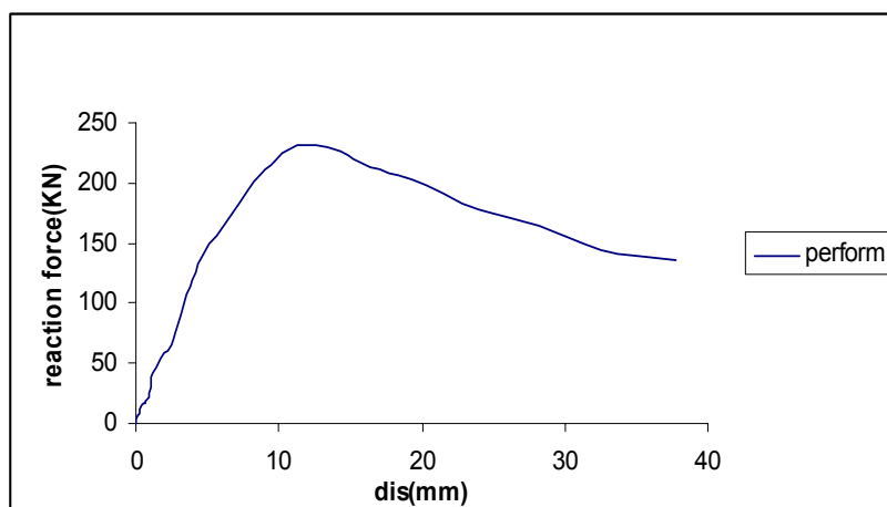
۷- نمودار پوش سیستم ترکیبی قاب خمشی تقویت شده با پانل پیش ساخته سبک
