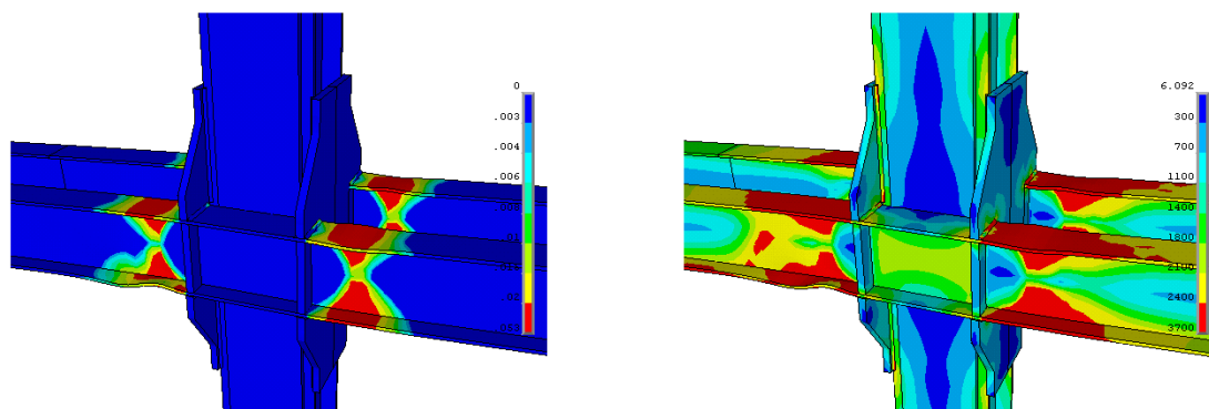
شکل ۱۴: توزیع تنش فون میسزو کرنش پلاستیک معادل در زاویه دریفت ۰/۰۵ رادیان در بارگذاری سیکلی، مدل KHV04 [۲]
