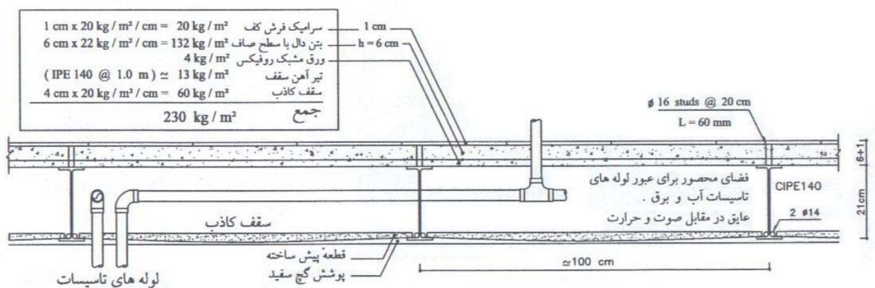
شکل ۱: وزن اجزای مختلف سقف مرکب بتنی با روفیکس
