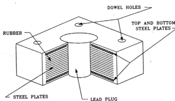
شکل: نشمینهای لاستیکی با هسته سربی
