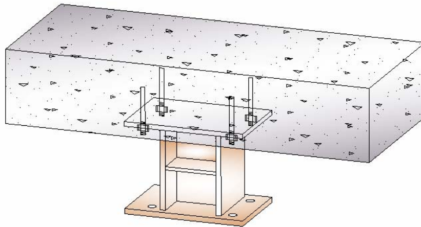
شکل ۸- نصب پانل برشی در سازه موجود
