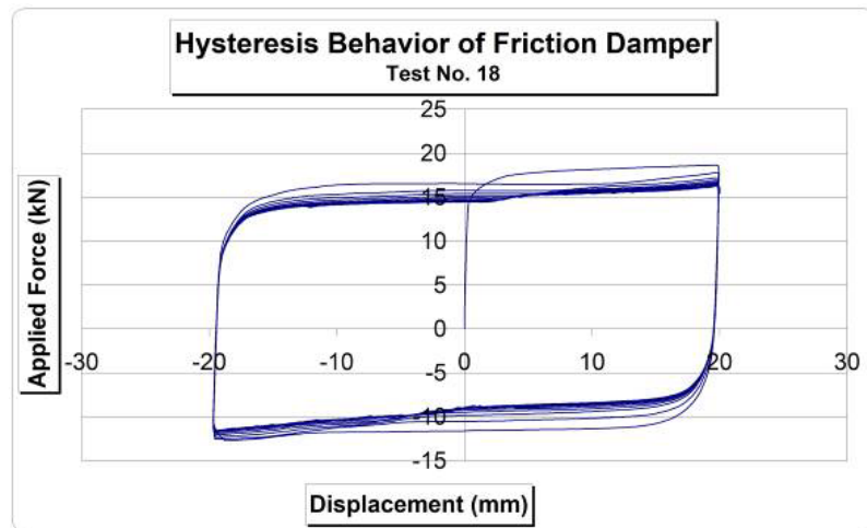
ج : اتصال ساندویچی (رفتار مناسب)
