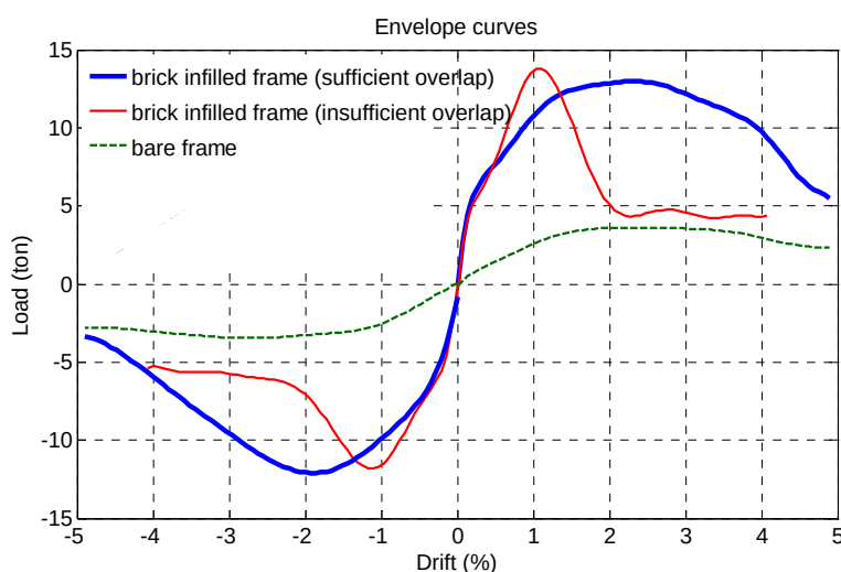
شکل 11: پوش منحنی هیستریزیس در نمونه‌های مختلف
