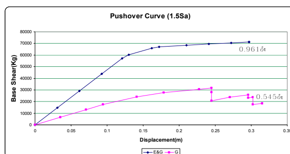
نمودار (۱): نمودار برش پایه-تغییر مکان دو قاب چهار طبقه در سطح زلزله طراحی ۲٪ در ۵۰ سال
