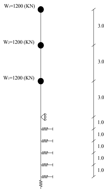
شکل ۹: مدل تحلیلی سه درجه آزادی سیستم مقاوم‌ساز نوین
