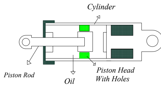
شکل (۱): میراگر مایع ویسکوز (Viscous fluid Damper)
