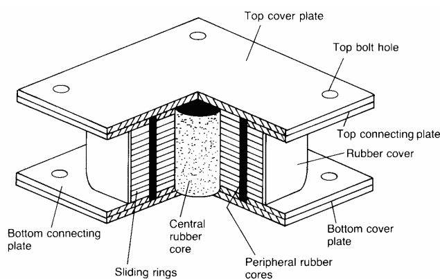
شکل: نشیمنهای جداسازی اصطکاکی پس جهنده
