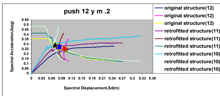
نمودار ۱۴- منحنی‌های ظرفیت و نیاز طیفی ساختمان ۱۲ طبقه قبل و بعد از تقویت (نقطه هدف) Y
