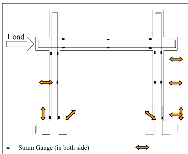
شکل 4: محل و تعداد ابزارهای اندازه‌گیری نصب شده روی نمونه‌ها
