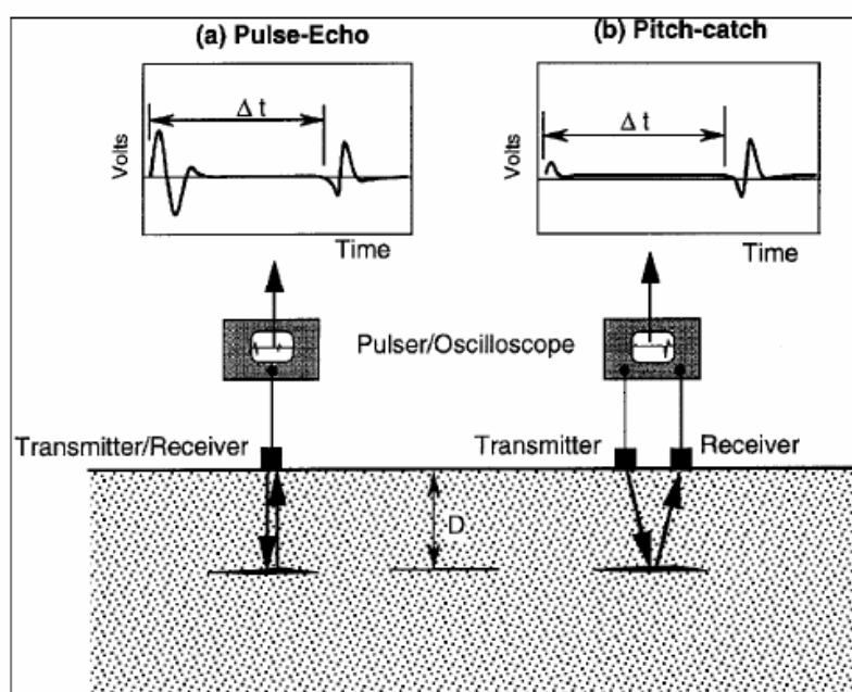
شکل (۱-۱): نحوه عملکرد روش‌های انعکاس ارتعاش و جلب ارتعاش
