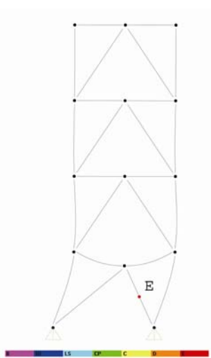
شکل ۱۰: توزیع مفاصل در انتهای تحلیل
