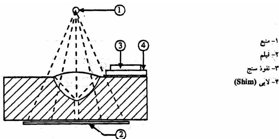
شکل (۲-۲): رادیوگرافی از جوش لب
