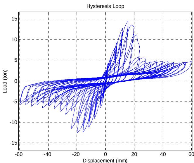
شکل ۹: منحنی رفتاری قاب با میانقاب آجر فشاری (با طول مهاری ناکافی در وصله آرماتورها)
