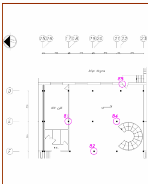
نقشه موقعیت سونداژ
