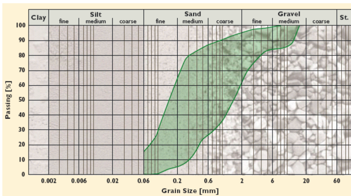
شکل ۵-۶ منحنی دانه بندی خاک تحت بهسازی
