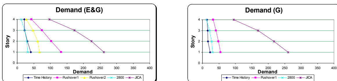
نمودار(۴): به ترتیب نمودار مقایسه‌ای تقاضای قاب چهار طبقه G و E&G در سطح زلزله طراحی ۱۰٪ در ۵۰ سال
