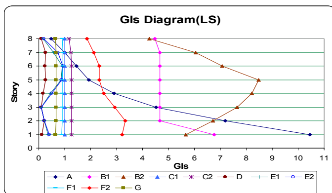
نمودار (۹): مقایسه شاخص‌های مقاومتی قاب E&G در سطح زلزله ۱۰٪ در ۵۰ سال
