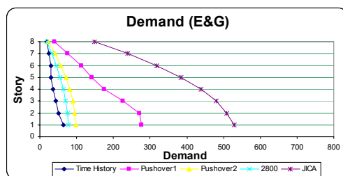
نمودار (۶): نمودار مقایسه‌ای تقاضای قاب هشت طبقه E&G در سطح زلزله طراحی ۱۰٪ در ۵۰ سال
