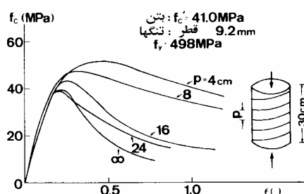
اثر محصور کنندگی بر مقاومت فشاری و شکل‌پذیری بتن
