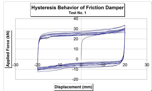
الف : سطوح تماس هموار (رفتار نسبتاً مناسب)
