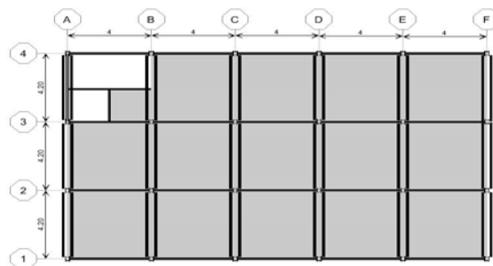
پلان ساختمان شماره ۱
