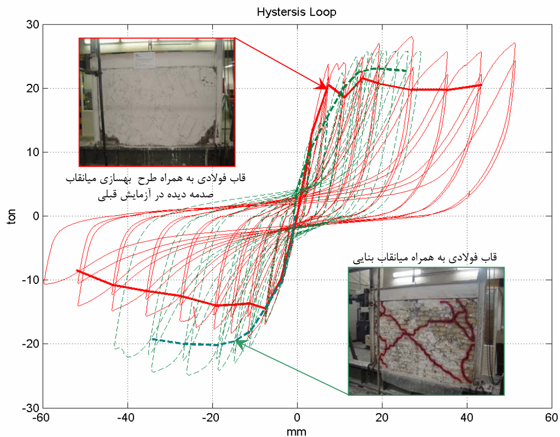
شکل ۱۱: منحنی هیستریزیس دو آزمایش
