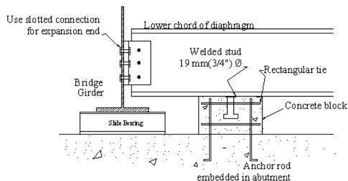
شکل : موقعیت ابزار مستهلک‌کننده‌ی انرژی در پل
