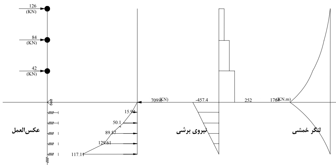
شکل ۱۰: توزیع نیروهای جانبی و نیروهای داخلی
