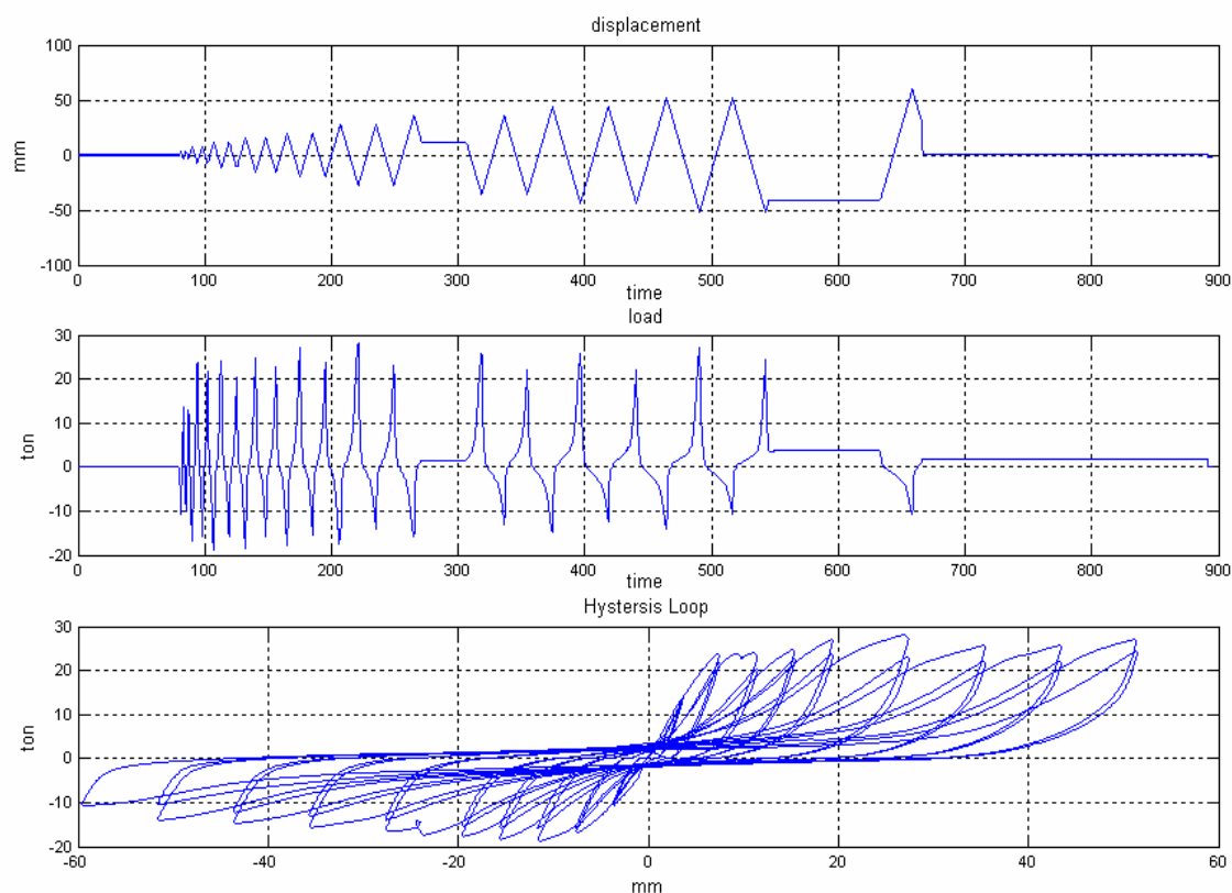
شکل ۹ منحنی اطلاعات خروجی جک
