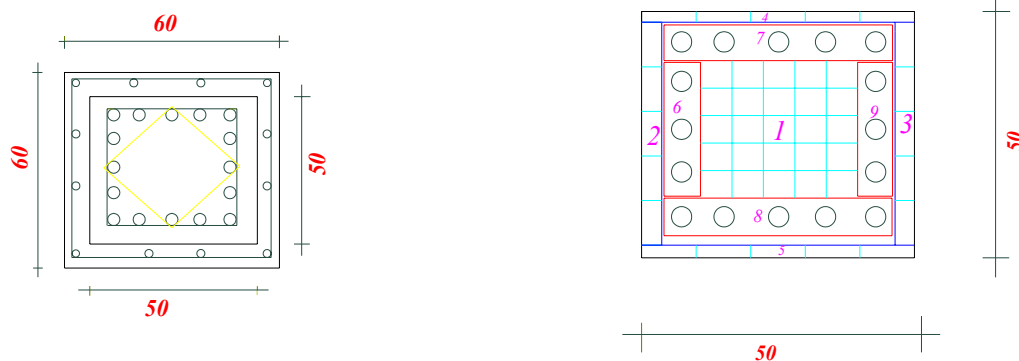
شکل (۴): نحوه‌ی مدل کردن مقطع در نرم افزار Open Sees
