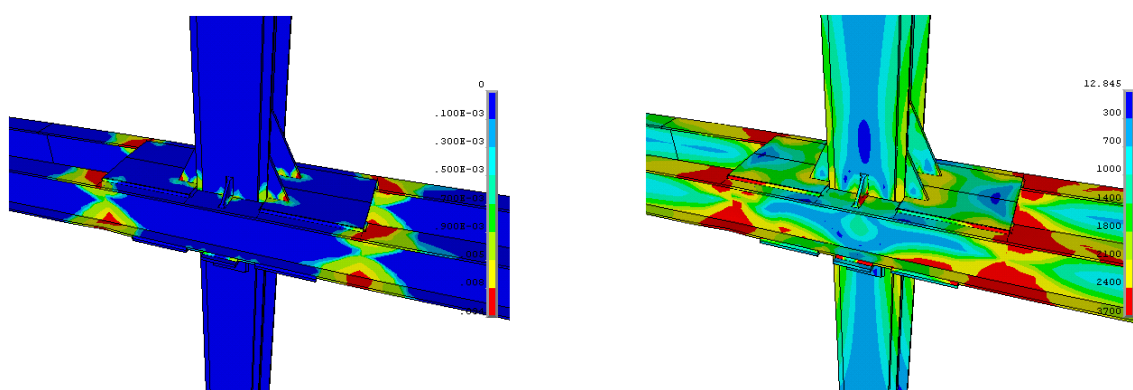
شکل ۱۲: توزیع تنش فون میسزو کرنش پلاستیک معادل در زاویه دریفت 0.3^\circ در بارگذاری سیکلی، مدل KHV02 [۲]
