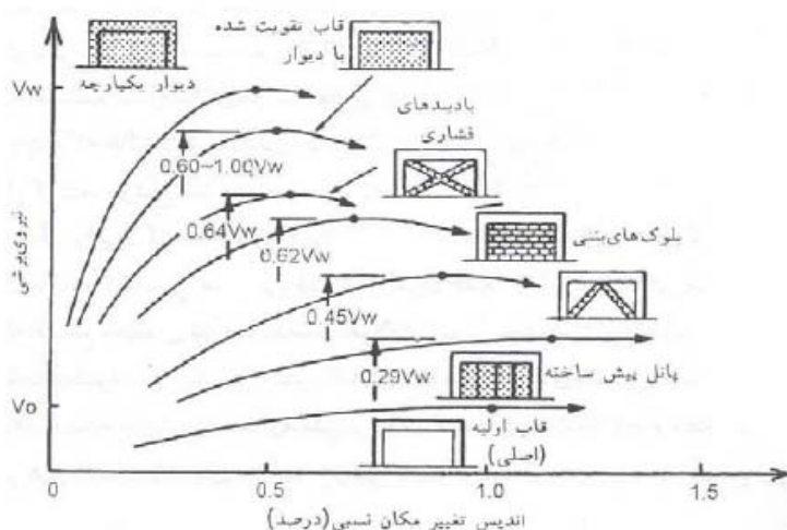
۳- نمودار بار - تغییر مکان نسبی برای قابهای تقویت شده با روشهای مختلف [7]
