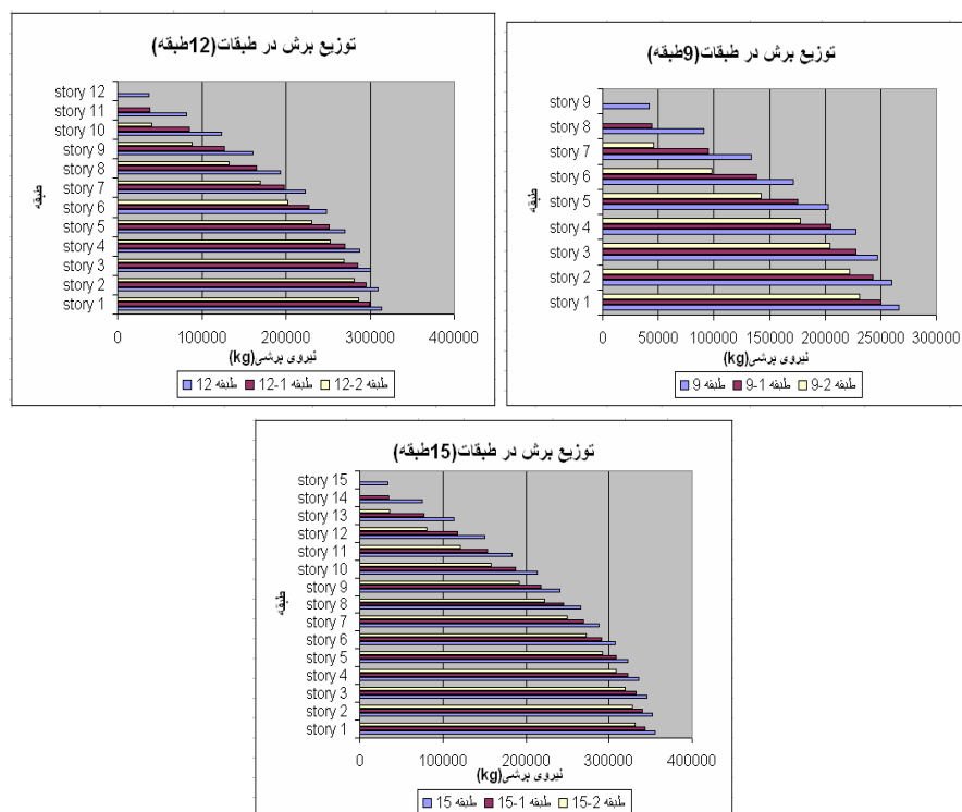
نمودار ۲- توزیع برش در ساختمان ۹ طبقه نمودار ۳- توزیع برش طبقات در ساختمان ۱۲ طبقه نمودار ۴- توزیع برش طبقات در ساختمان ۱۵ طبقه
