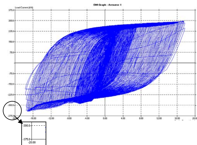
ب) نمودار هیستریزیس (واحد ها بر حسب کیلو نیوتن)
