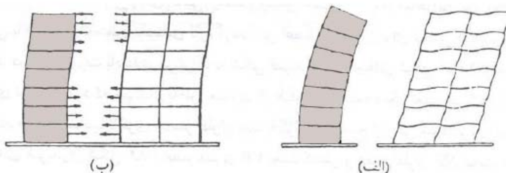
۴- تغییر شکل قاب خمشی و پانل پیش ساخته سبکو سیستم ترکیبی آنها
