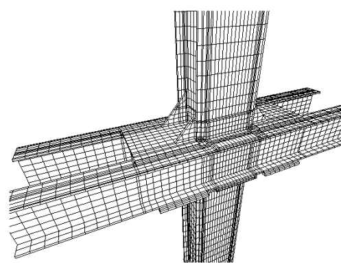
شکل ۳: مدل اجزای محدود نمونه آزمایشگاهی
