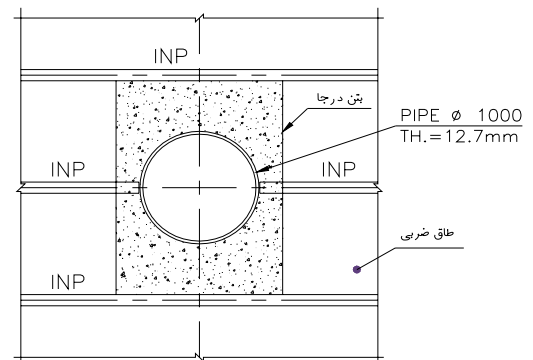
شکل ۴: پلان سیستم مقاوم ساز در طبقات
