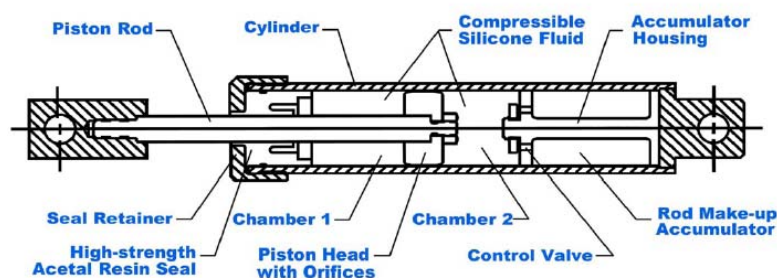
شکل : میراگر ویسکوز مایع
