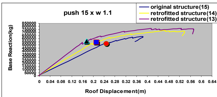
نمودار ۷- منحنی ظرفیت ساختمان ۱۵ طبقه قبل و بعد از تقویت (در جهت X)
