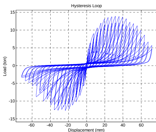
شکل 8: منحنی رفتاری قاب با میانقاب آجر فشاری (با طول مهاری کافی در وصله آرماتورها)
