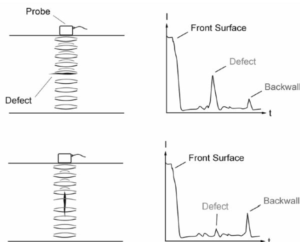
شکل ۳: انعکاس امواج فشاری در برخورد با نقایص موجود
