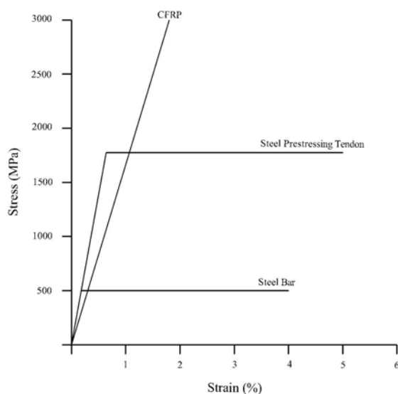
شکل ۳- نمودار تنش-کرنش برای فولاد و CFRP [۱۳]
