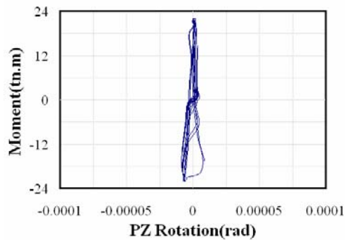
ب. مدل KHV02
