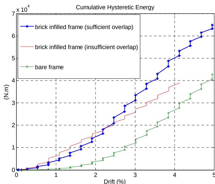
شکل 12: منحنی انرژی هیستریزیس تجمعی در نمونه‌های مختلف
