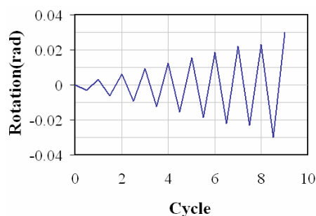
شکل ۴: دوران اعمالی به اتصال ساخته شده در مرکز تحقیقات مسکن [۶]
