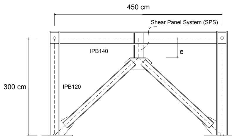
شکل ۱- مشخصات کلی قابها
