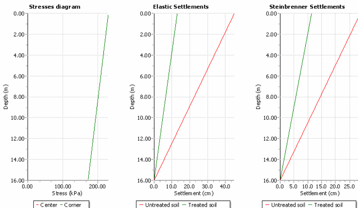
شکل ۶-۸. توزیع تنش و نشست‌های محاسبه شده در زیر پی
