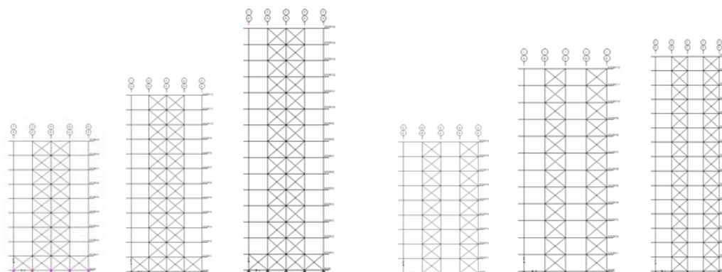
الف- در جهت X ب- در جهت Y شکل ۱- آرایش بادبندی ساختمان‌های ۹-۱۲-۱۵ طبقه
