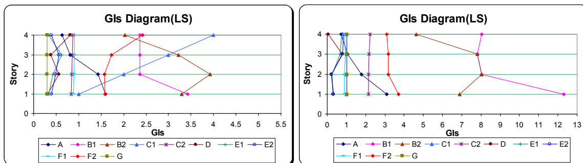
نمودار (۷): مقایسه شاخص‌های مقاومتی قاب G ..... قاب E&G در سطح زلزله ۱۰٪ در ۵۰ سال
