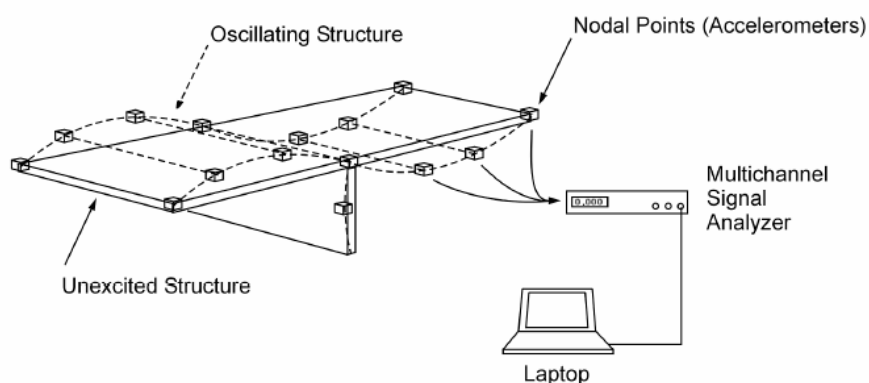
شکل ۶: تحلیل مودال اعضائی یک سازه در مقیاس بزرگ
