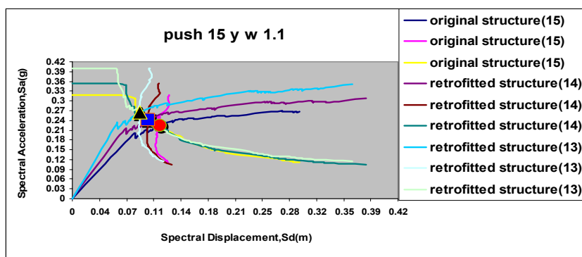
نمودار ۱۰- منحنی‌های ظرفیت و نیاز طیفی ساختمان ۱۵ طبقه قبل و بعد از تقویت (نقطه هدف) Y
