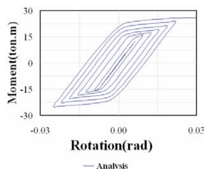
شکل ۵: منحنی چرخه‌ای ممان-دوران مدل اجزای محدود نمونه آزمایشگاهی [۲]
