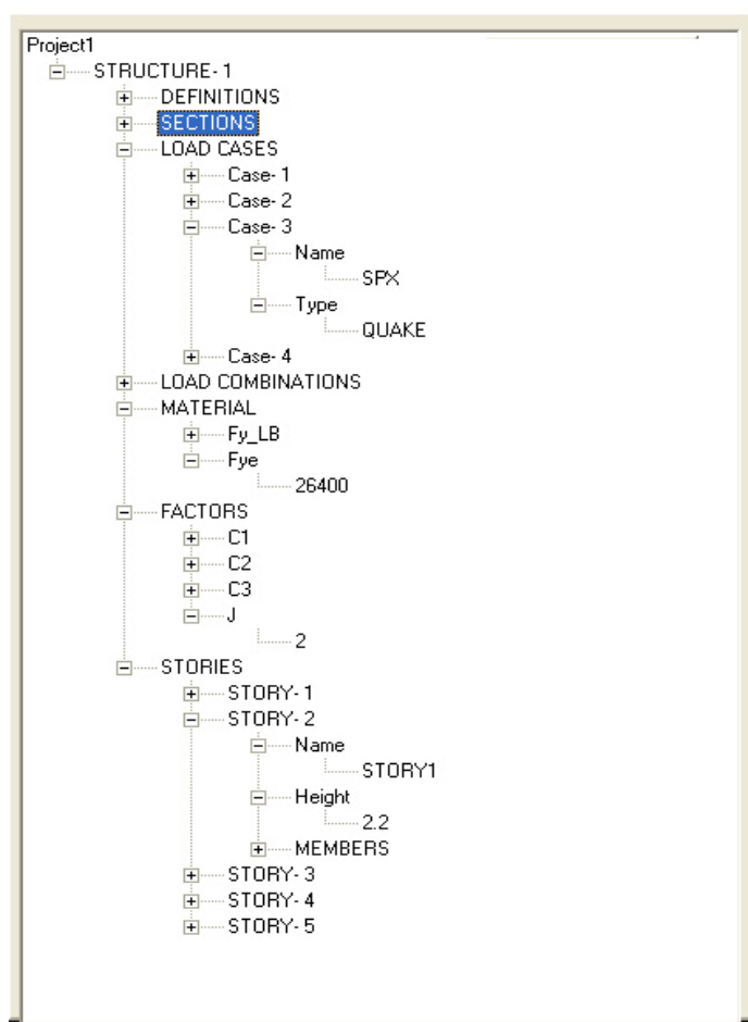
شکل ۲- بخشی از ساختار گسترش یافته کلاس Structure
