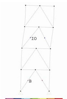
شکل ۱۳: توزیع مفاصل در انتهای تحلیل ( \delta_t = 7 \text{ cm} )
