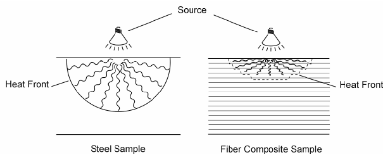
شکل ۴: هدایت گرمایی در نمونه‌های فولادی و کامپوزیتی
