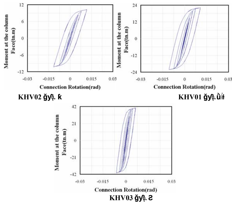
شکل ۱۷. منحنی‌های لنگر چرخش اتصال [۲]
