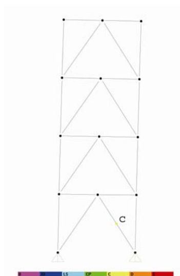
شکل ۹: نمایش اولین مفصلی که از ناحیه L_s عبور کرده است
