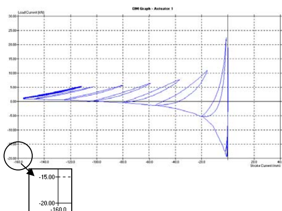
ب) نمودار هیستریزس (واحد ها بر حسب کیلو نیوتن)
