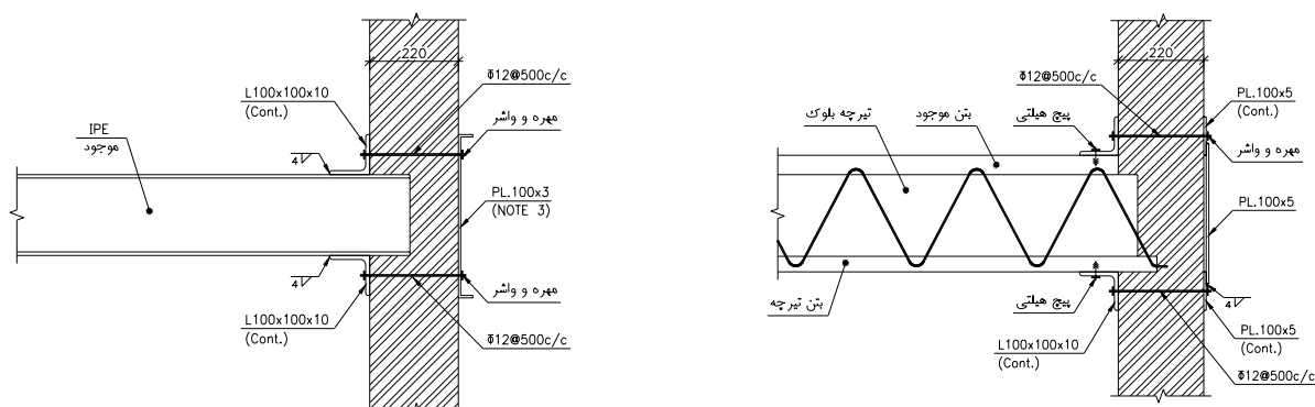
شکل ۷: جزئیات اتصال سقف‌ها به دیوارها
