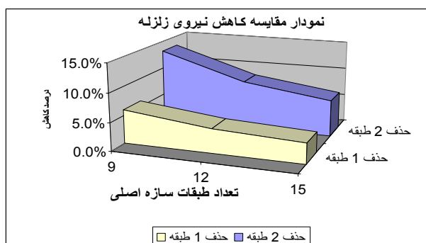
نمودار ۶- مقایسه کاهش نیروی زلزله با حذف طبقه برای مدل های ساختمانی مختلف
