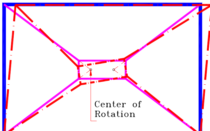
ب: تشکیل مراکز آنی دوران شکل ۲: ساز و کار رفتار مهاربند اصطکاکی
