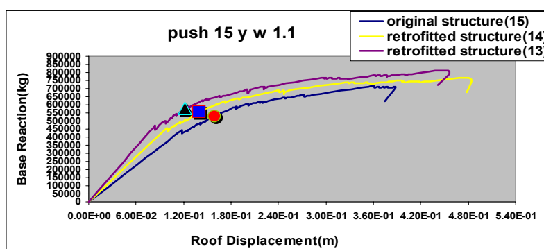
نمودار ۹- منحنی ظرفیت ساختمان ۱۵ طبقه قبل و بعد از تقویت (در جهت Y)
