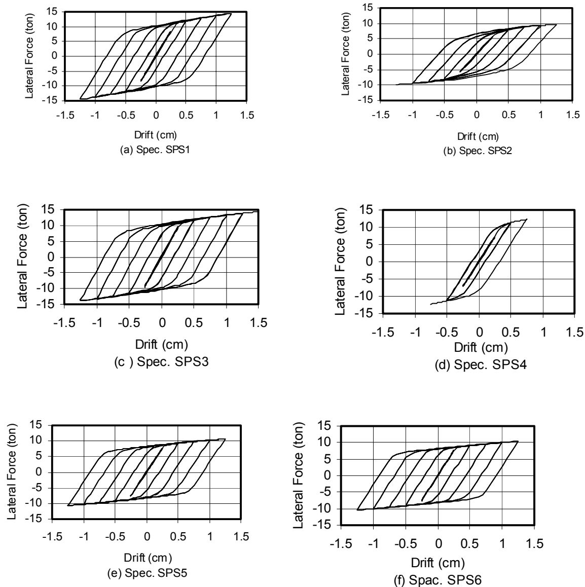
شکل ۴- پاسخ هیستریک نیرو-جابجایی جانبی قابها
