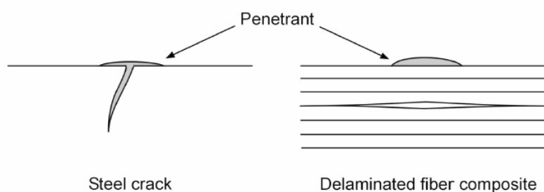
شکل ۲: تفاوت نفوذ مایع در فولاد و لایه‌های کامپوزیت
