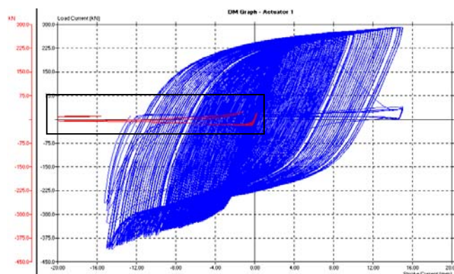
شکل ۵: مقایسه نمودار هیستریزیس عضو معمولی و مقاوم در برابر کماتش [۳]
