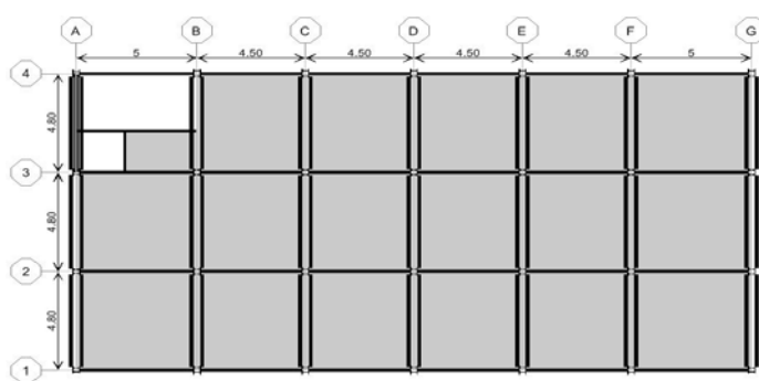
پلان ساختمان شماره ۳
