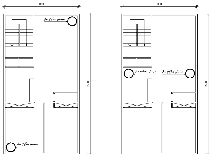
شکل ۱: جانمایی مختلف سیستم سازه‌ای بهسازی در پلان ساختمان
