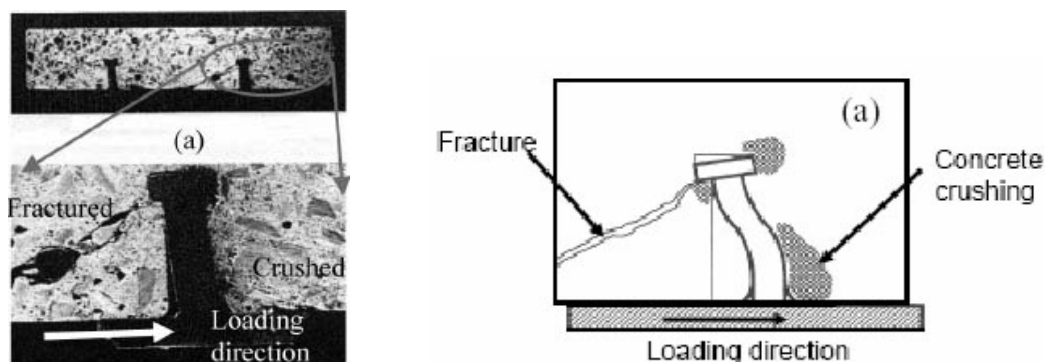
شکل : شکست بتن در مجاورت گل‌میخ
