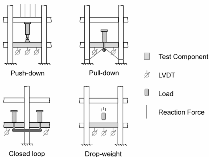
شکل ۷: مکانیزم معمول بارگذاری در روش بارگذاری سریع
