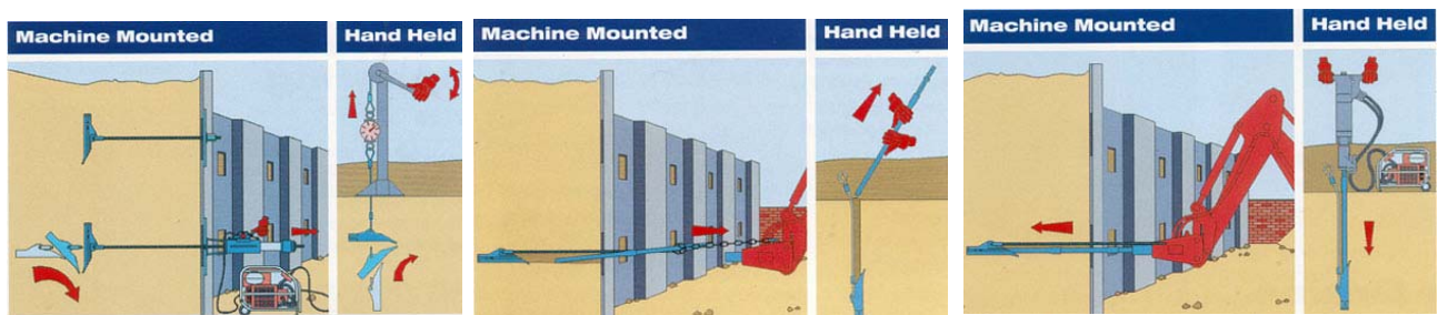
(شکل ۳-۳) روش نصب قلاب داکبیل برای توده‌های خاکی سنگین تر با استفاده از پیکور و یا چکش تخریب دستی
