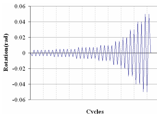
شکل ۱۰: بارگذاری سیکلی اعمالی به نمونه‌ها
