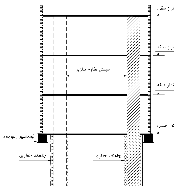
شکل ۲: جانمایی سیستم سازه‌ای بهسازی لرزه‌ای در ارتفاع ساختمان مفروض
