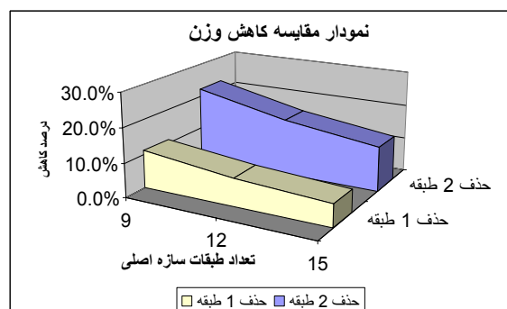
نمودار ۵- مقایسه کاهش وزن با حذف طبقه برای مدل های ساختمانی مختلف
