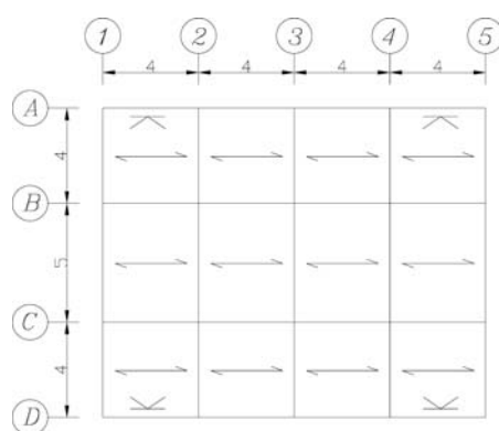
شکل ۶: سازه مورد بررسی
