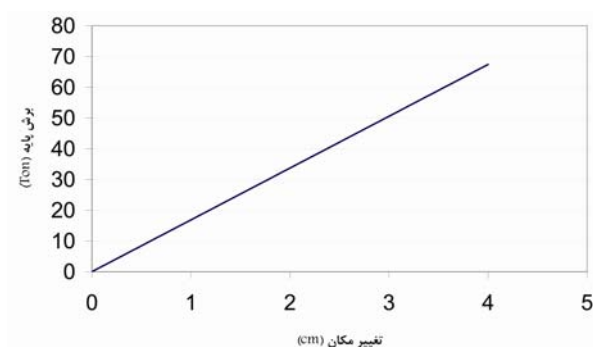
شکل ۱۱: نمایش منحنی ظرفیت سیستم مهاربند مقاوم در برابر کماتش در سطح خطر ۱
