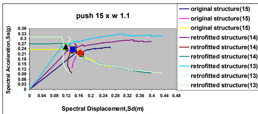
نمودار ۸- منحنی های ظرفیت و نیاز طیفی ساختمان ۱۵ طبقه قبل و بعد از تقویت (نقطه هدف) X
